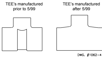
FIG. 5 GRINNELL TEE
